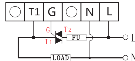
ZKD-2A-II调整器接线图
