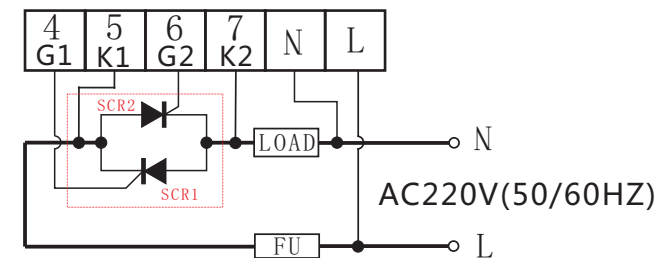
ZKD-3A-II调整器接线图
