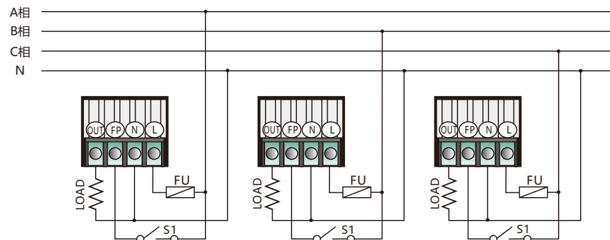
三相接线图：
