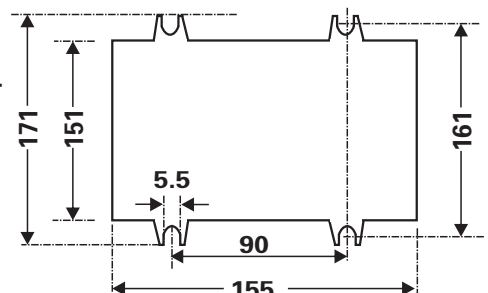
图2:底部平面图尺寸
