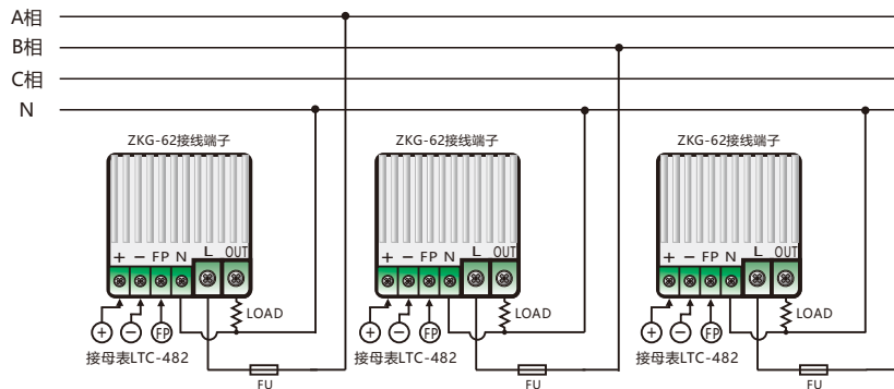
三相接线图：
