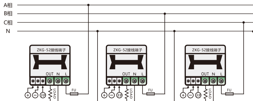
三相接线图：
